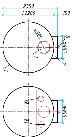
Вид А
